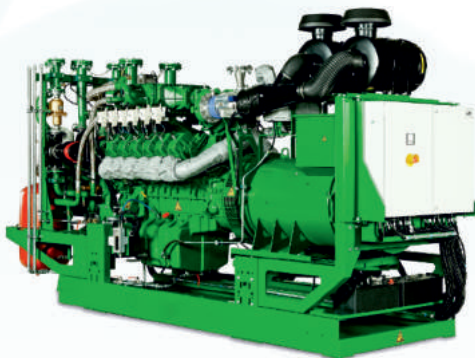
Warmtekrachtkoppeling-generator (WKK)
